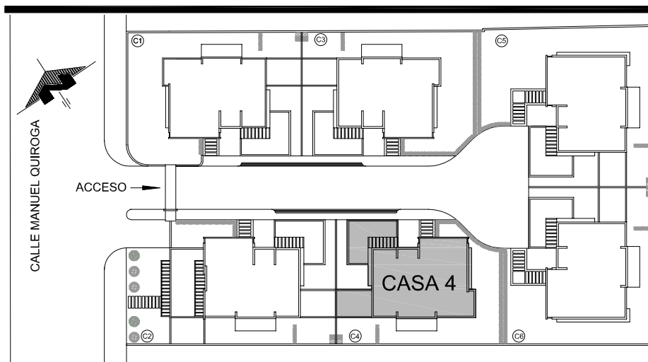
IMPLANTACION
