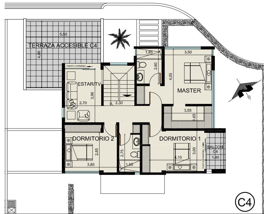
PLANTA ALTA
