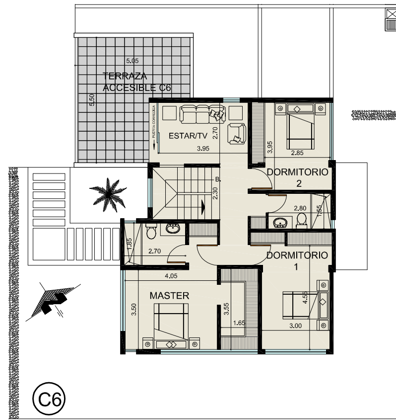
PLANTA ALTA
